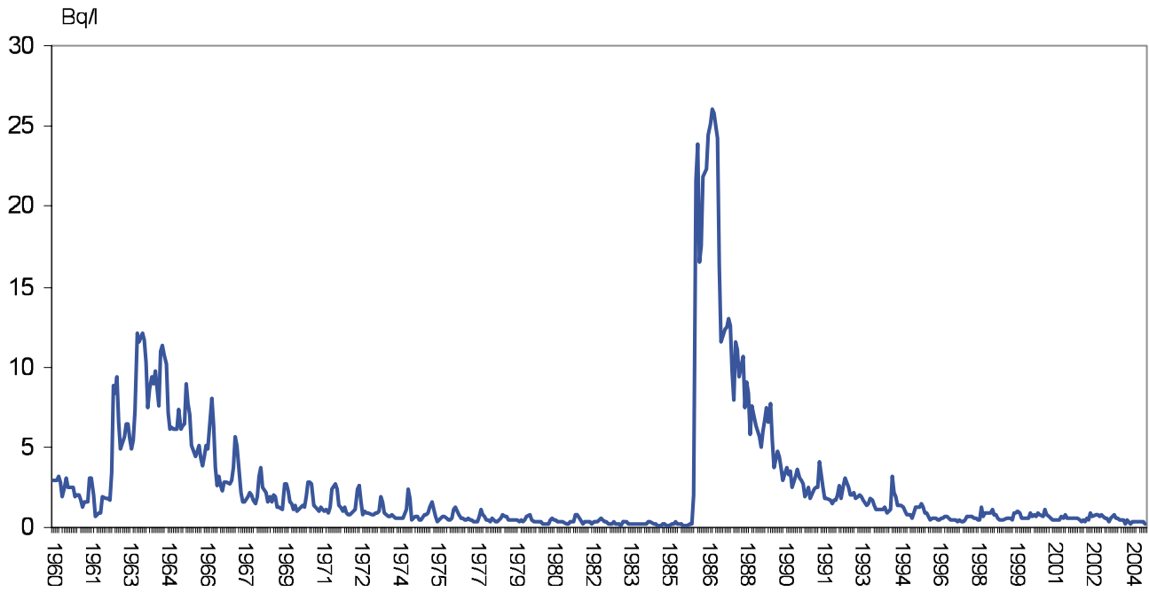
Kuva 8.2. Maidon keskimääräinen 137 Cs-pitoisuus Etelä-Suomessa tuotetussa maidossa vuodesta 1960 lähtien. Bild 8.2. Genomsnittlig halt av 137 Cs i mjölk producerats i Södra Finland sedan 1960. Fig. 8.2. 137 Cs in milk (Bq/l) in Southern Finland since 1960.
