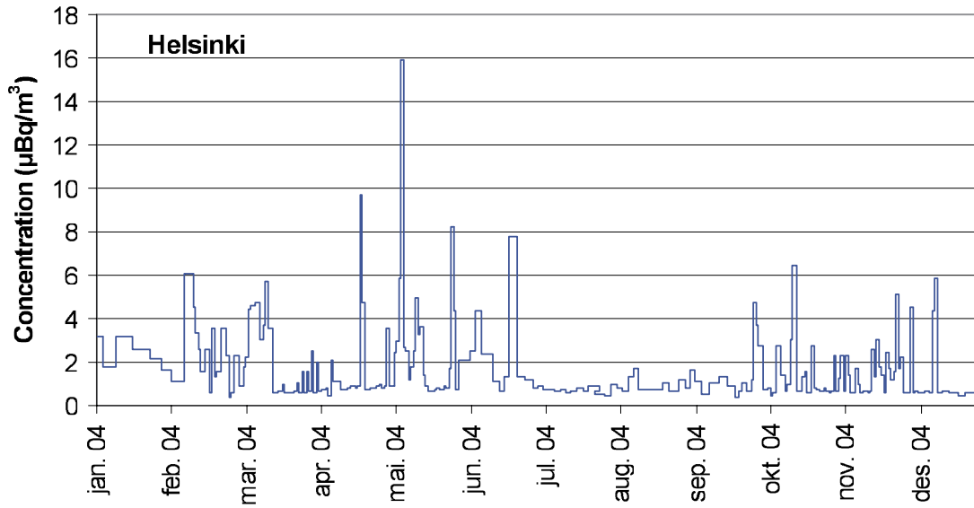
Kuva 3.4. Ilman ^{137}\text{Cs} -pitoisuuden vuorokausikeskiarvot Helsingissä vuonna 2004.
