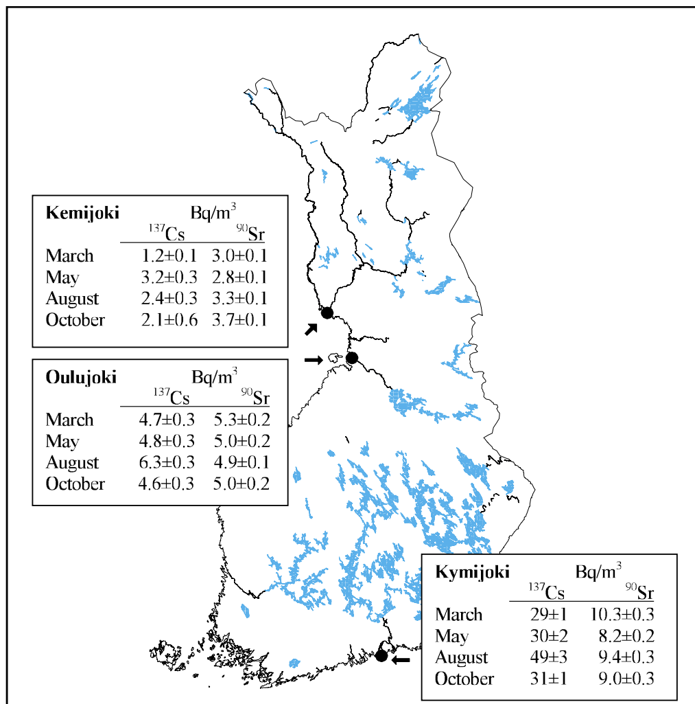
Kuva 6.1. Pintaveden näytteenotuspisteet ja näytteiden 137 Cs- ja 90 Sr-pitoisuudet (Bq/m 3 ) vuonna 2004.
