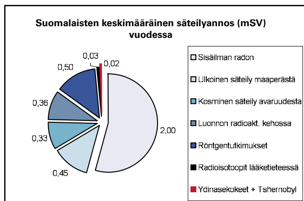
Kuva 1.1. Suomalainen saa ionisoivasta säteilystä keskimäärin 3,7 millisievertin säteilyannoksen vuodessa. Tässä raportissa esitettävät säteilyaltistuksen lähteet aiheuttavat yhteensä noin 0,7 % osuuden koko annoskasta (punainen siivu kuvassa).
