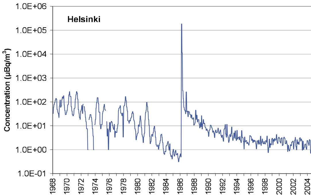
Kuva 3.5. Ilman ^{137}\text{Cs} -pitoisuus Helsingin seudulla vuosina 1968–2004. Ennen Tshernobylin onnettomuutta (v. 1986) esiintyvä ^{137}\text{Cs} on peräisin ilmakehässä tehdyistä ydinasekokeista. Tälle laskeumalle on tyypillistä kuvassa näkyvä vuodenaikaisvaihtelu.
