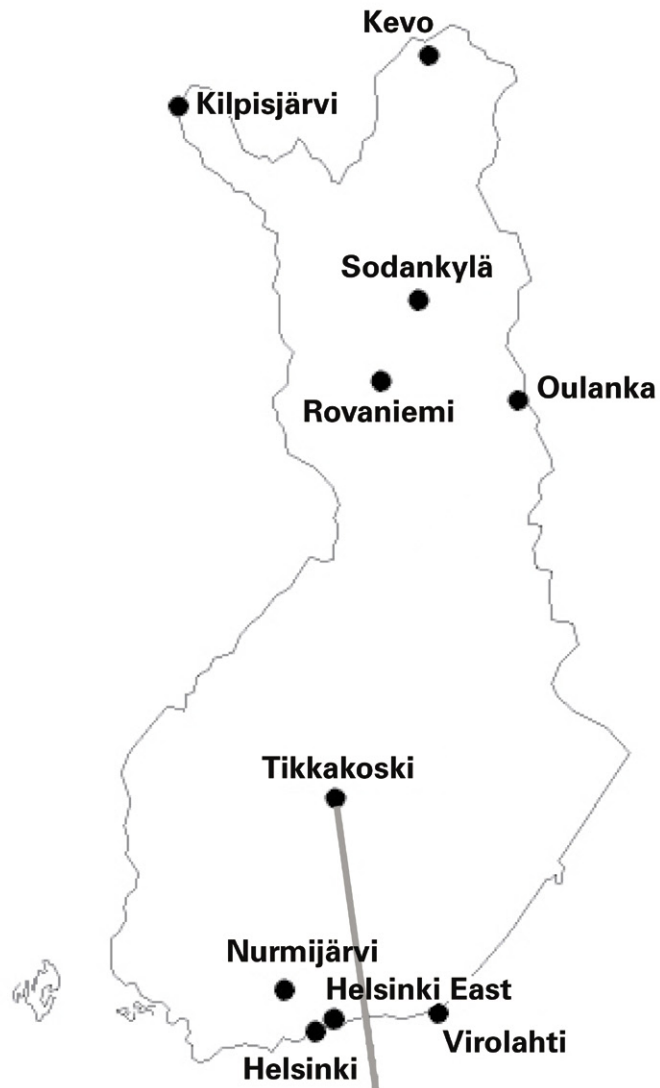
Kuva 4.1. Seuranta-asemat vuonna 2004. Bild 4.1. Bevakningsstationerna år 2004. Fig. 4.1. Monitoring stations in 2004.
