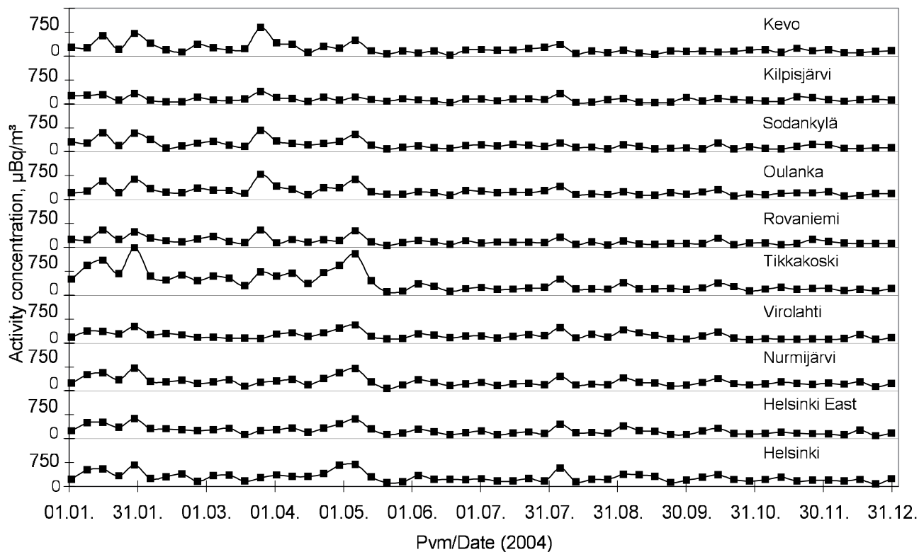
Kuva 4.2. Aerosolin pitkäkäisen beeta-aktiivisuuden pitoisuudet mikrobecquerelliä kuutiometrissä ilmaa ( \mu\text{Bq}/\text{m}^3 ) v. 2004.
