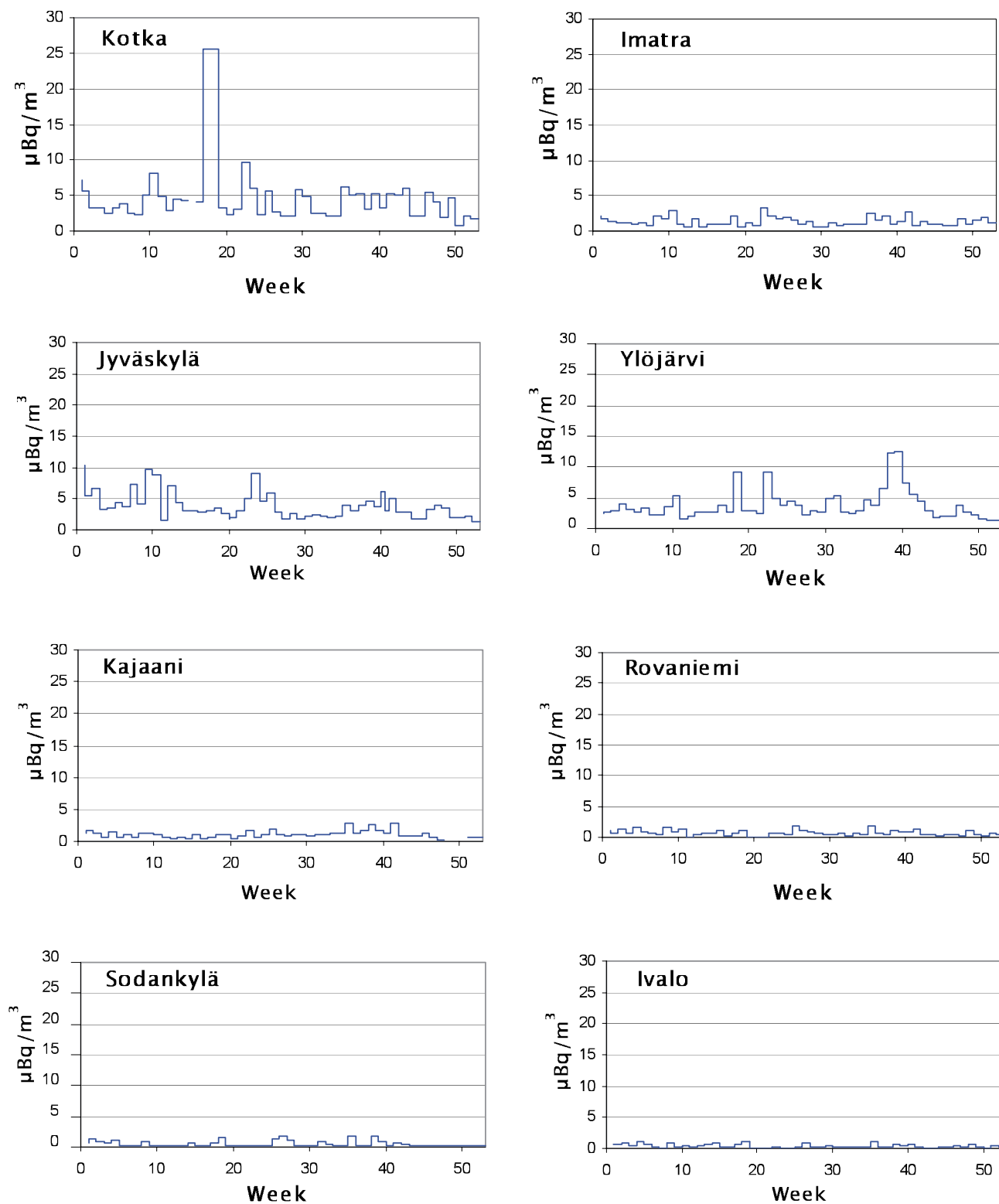
Kuva 3.3. ^{137}\text{Cs} -pitoisuuksien viikkokeskiarvot ulkoilmassa eri valvonta-aseilla vuonna 2004.
