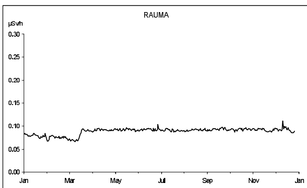
Kuva 2.3. Ulkoisen säteilyn annosnopeus kahdeksalla mittausasemalla vuonna 2004.
