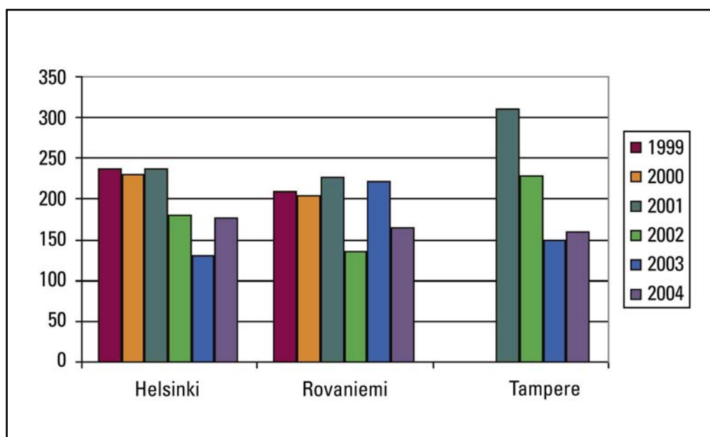
Kuva 10.2. Kehossa oleva keskimääräinen Cs-137 sisältö vuoden 2004 loppupuolella. Ryhmissä on mukana kaikki yli 14-vuotiaat, jotka kävivät mittauksessa. Bild 10.2. Kroppsinnehållet av Cs-137 som medelvärde för kvinnor och män i slutet av 2004. I grupperna ingår alla personer äldre än 14 år. Fig 10.2. The Cs-137 body content as mean for women and men at the end of 2004. All persons older than 14 years are included in the groups.
