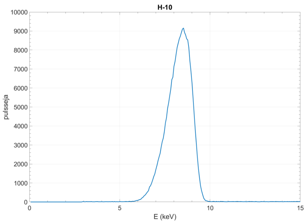
Kuva 9. E_{\text{mean}} = 8,18 keV, FWHM=1,67 keV.
