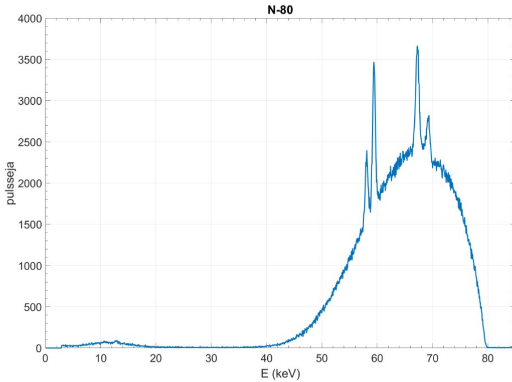
Kuva 8. E_{\text{mean}} = 64,73 keV, FWHM=20,71 keV. Mitattu 320 kV putkella.
