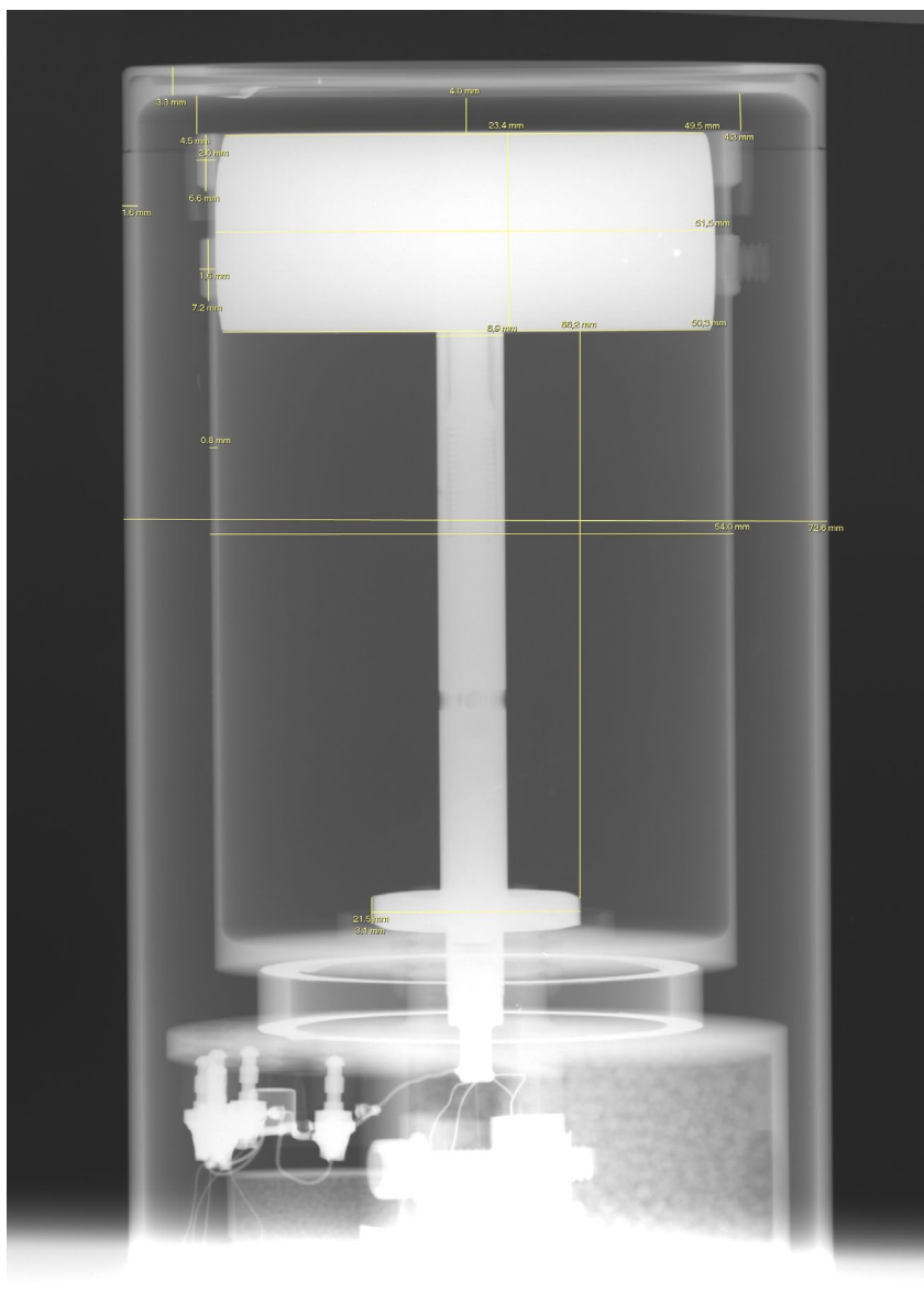
Kuva 1. Röntgenkuva ilmaisimesta. Kuvassa näkyy Carestream Vue PACS ohjelmalla mitatut dimensiot. Mittakaava saatiin end capin halkaisijan avulla.
