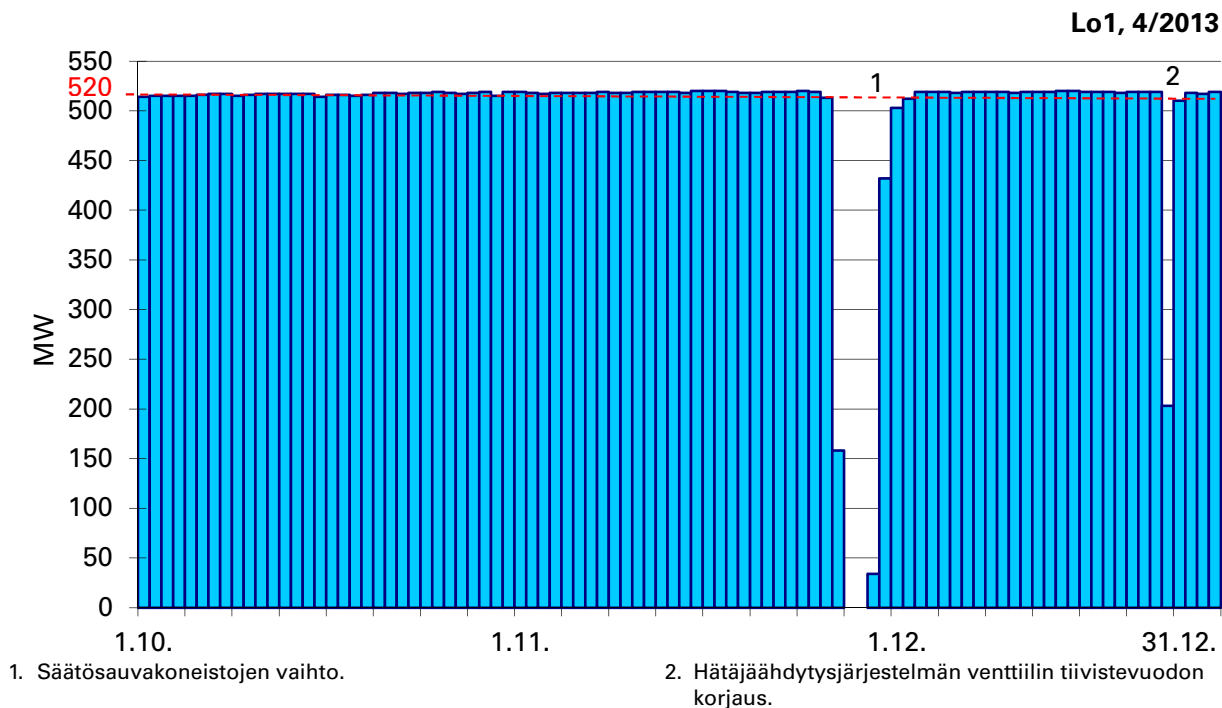
Kuva 1. Loviisa 1:n keskimääräinen vuorokautinen bruttosähköteho loka–joukukuussa 2013.
