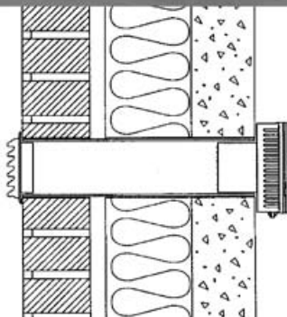
Kuva 10.3. Seinään asennettava ulkoilmaventtiili.
