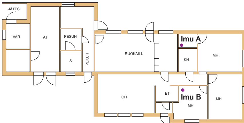
Kuva 4.7. Imupisteiden sijainti pientalossa, jossa kantava väliseinä jakaa pohjalaatan kahteen erilliseen lohkoon.
