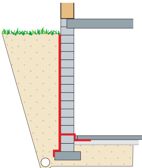
Kuva 14.2. Harkkorakenteisen kellariseinän radontorjunta RT-ohjekortin RT 81-10791 mukaisesti.
