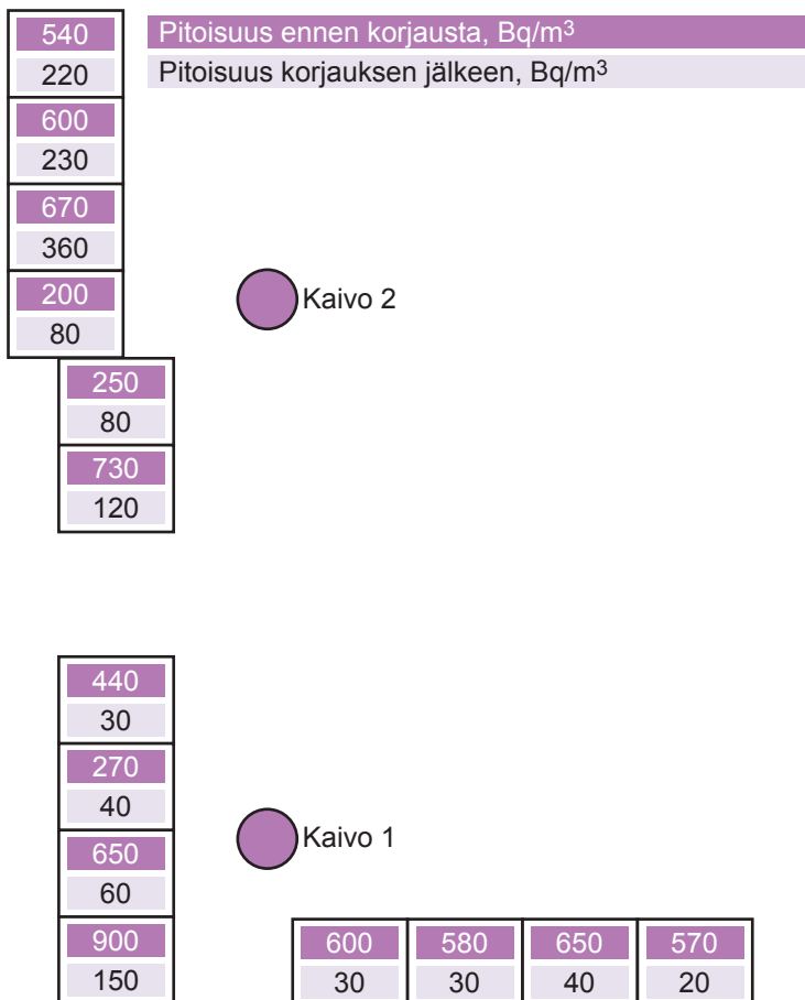
Kuva 5.4. Rivitaloyhtiön radonkaivojen sijoitus ja radonpitoisuuden muutokset asunnoissa.
