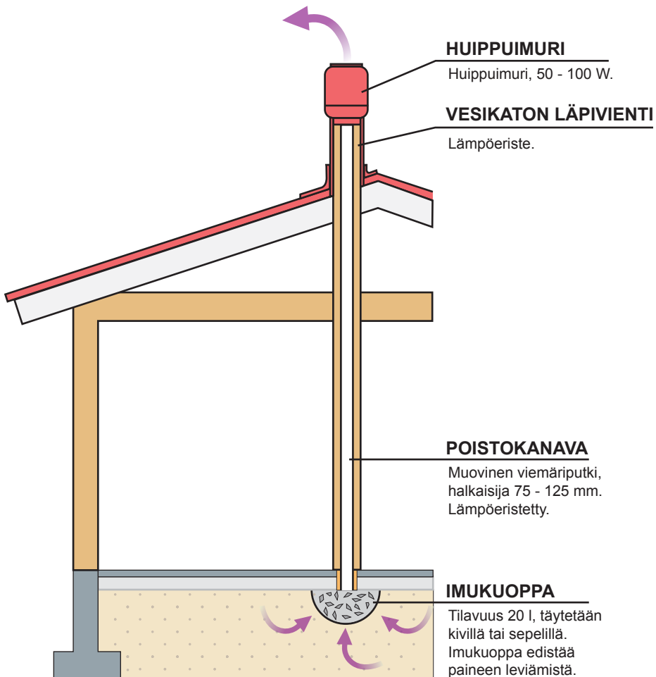
Kuva 4.2. Radonimurin toimintaperiaate ja rakenneosat.
