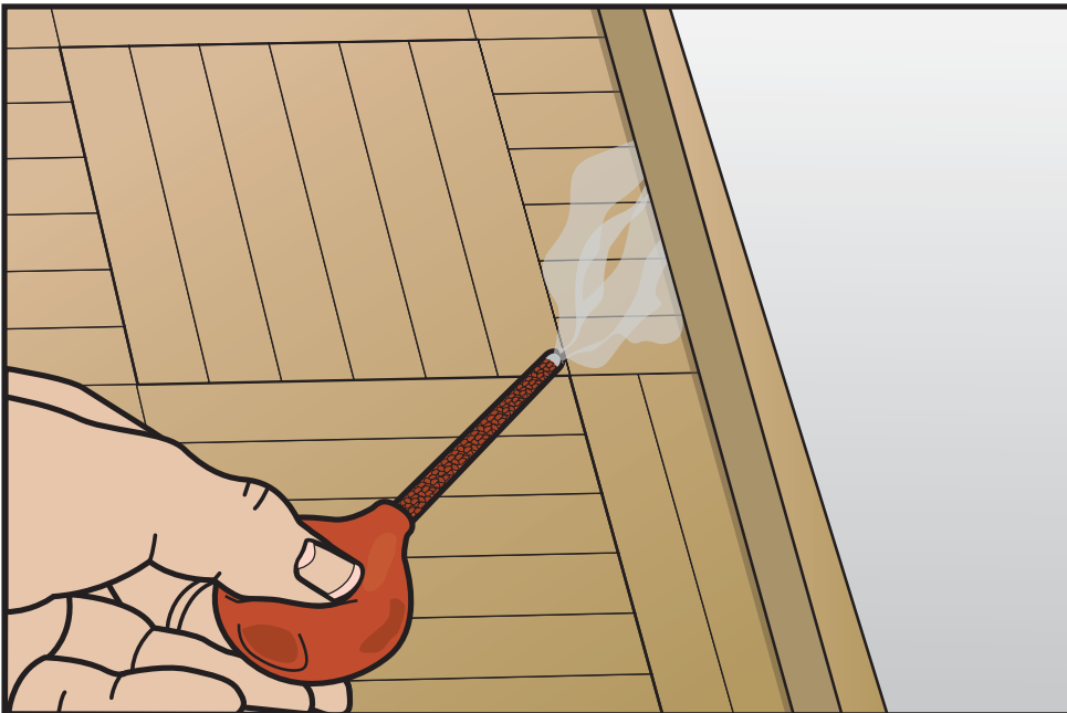
Kuva 12.3. Merkkisavulaitteen käyttöä lattialaatan ja sokkelin välisen raon ilmavirran havaitsemisessa. Kuvan esimerkissä asunnossa oli radonimuri ja merkkisavu virtasi raon kautta lattialaatan alle.
