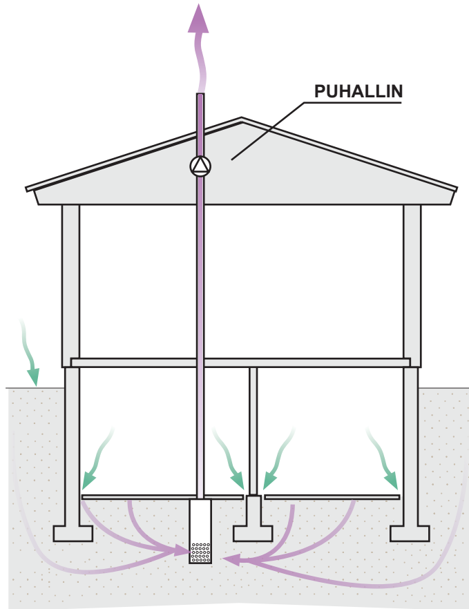
Kuva 4.5. Radonimuri kellarillisessa talossa, jossa on monilohkoinen alapohja. Imuri on toteutettu ns. syvällä imupisteellä. Maaperä on läpäisevää myös anturatasen alapuolella. Imupisteen vaikutus ulottuu koko rakennusalalle.
