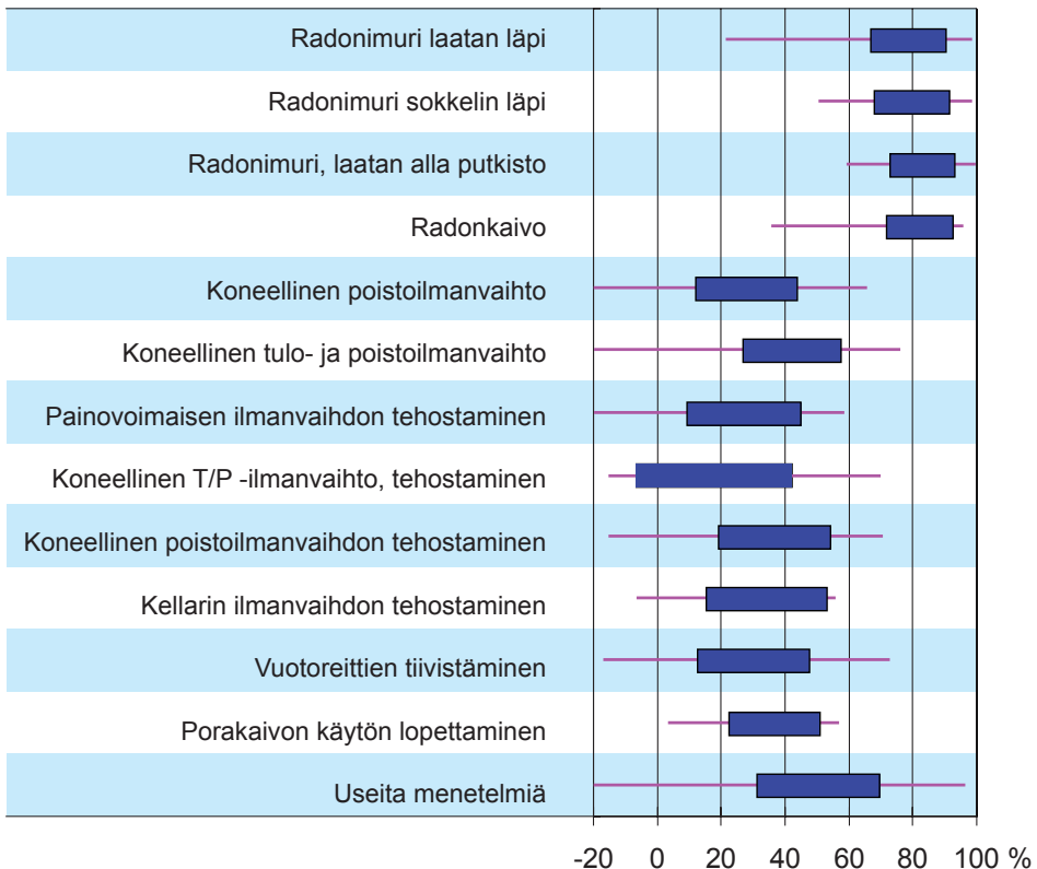
Kuva 2.1. Tyypillinen eri menetelmillä saavutettu radonpitoisuuden prosentuaalinen alenema (paksunnettu viiva, rajoina 25 % ja 75 % aineistosta) sekä vaihtelualue (ohut viiva). Negatiiviset arvot kertovat radonpitoisuuden luonnollisesta vaihtelusta kahdessa eri mittauksessa, kun alenema on alhainen.
