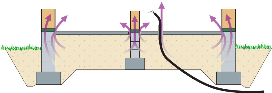
Kuva 1.2. Radonpitoisen ilman vuotoreittejä maanvaraisen laatan perustuksessa.
