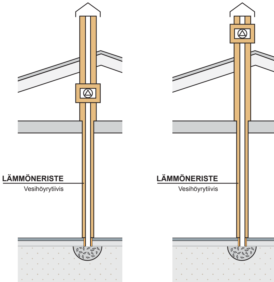
Kuva 4.10. Poistopuhaltimen sijoittaminen ja poistokanavan lämmöneristys.
