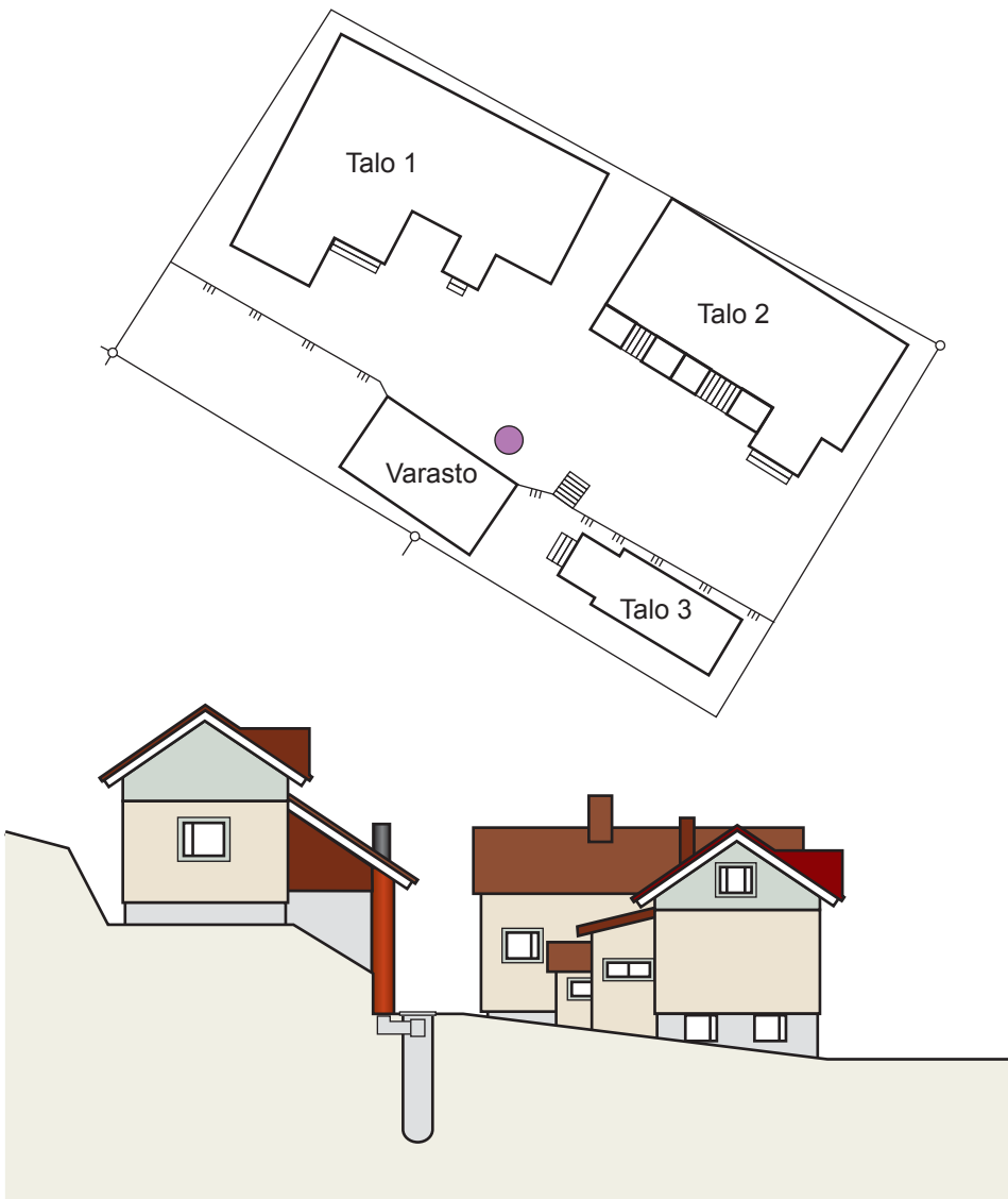
Kuva 5.10. Radonkaivon sijainti Pispalanharjulla olevan taloyhtiön pihalla.
