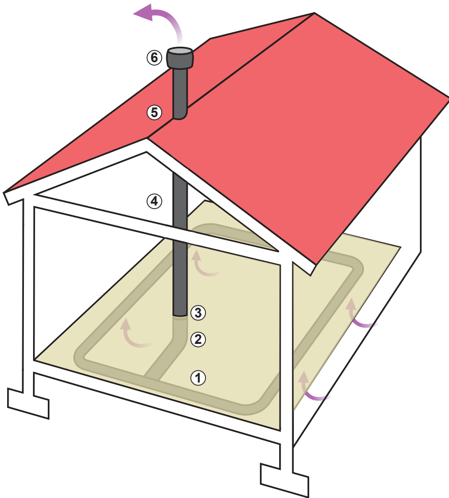
Kuva 14.4. Radonputkiston asentaminen maanvaraisen lattialaatan alle.
