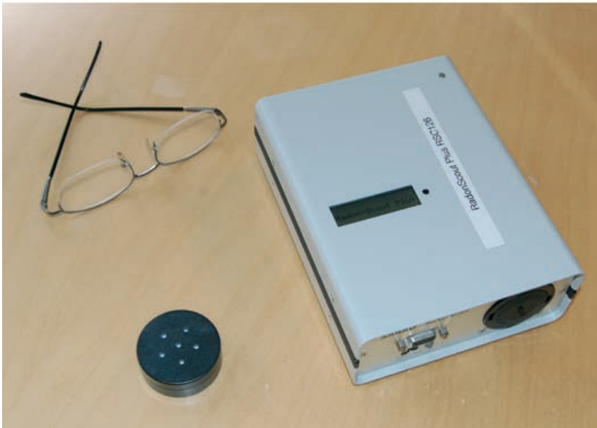
Kuva 12.1. Jatkuvasti toimivia radonmittalaitteita sekä postitse toimitettava radonmittauspurkki, jota käytetään radonpitoisuuden pitkän ajan keskiarvon määrittämiseen.
