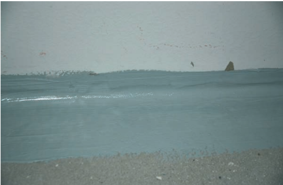
Kuva 6.3. Vuotavan lattiarakon tiivistäminen vedeneristysmassalla ja -nauhalla.
