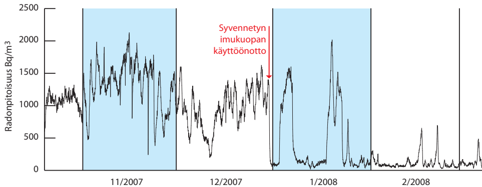
Kuva 4.12. Imupisteen syventämisen vaikutus radonpitoisuuteen tamperelaisessa omakotitalossa.
