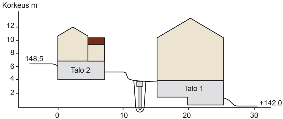
Kuva 5.12. Pispalanharjulla sijaitsevat rakennukset ja radonkaivon sijainti.
