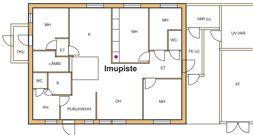
Kuva 4.6. Imupisteen sijainti yhtenäisellä suorakaiteen muotoisella laatalla varustetussa rivitaloasunnossa (A) ja pientaloasunnossa (B).
