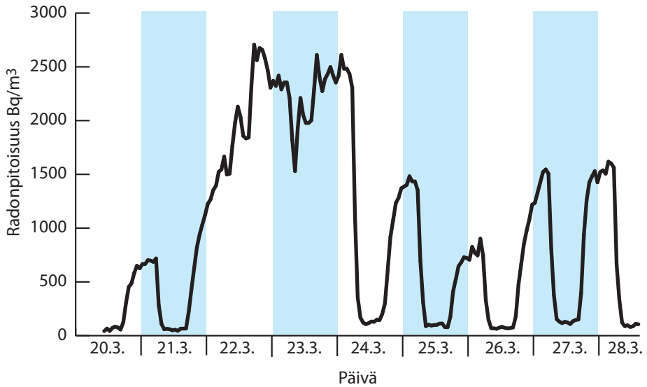
Kuva 11.3. Radonpitoisuuden voimakasta vaihtelua työpaikalla päivä- ja yöaikana.
