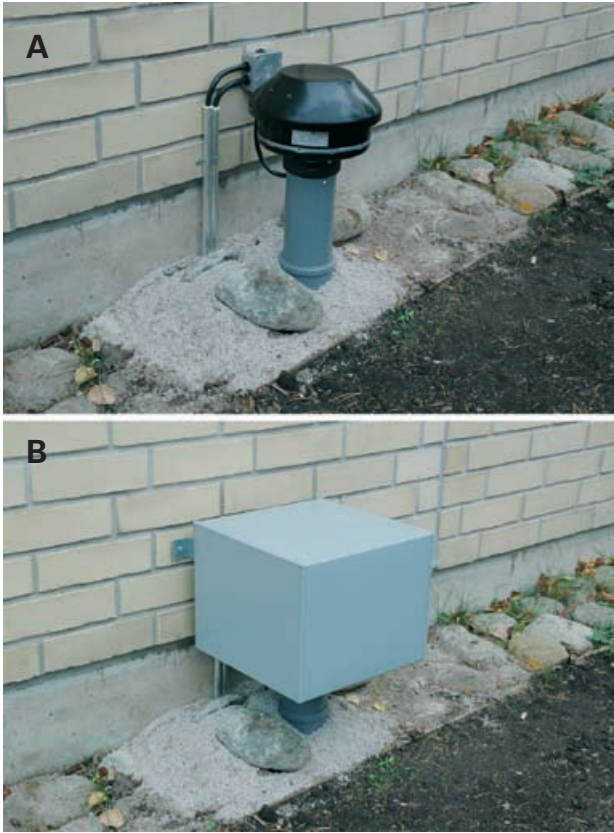
Kuva 10.6. Sokkelin viereen asennettu poistopuhallin (A) ja puhaltimen ympärillä oleva tehokas äänenvaimennin (B).
