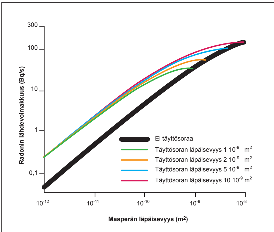
Kuva 1. Radonin virtausnopeus kellarilliseen asuntoon. Perusmuurin ja laatan välinen rako on 3 mm. Radonpitoisuus syväällä maaperän huokosilmassa on 37 000 Bq/m 3 . Täyttösoran paksuus laatan alla 15 cm. Paine-ero ulkoilmaan nähden kellarissa on 5 Pa. (Revzan ja Fisk, 1992)
