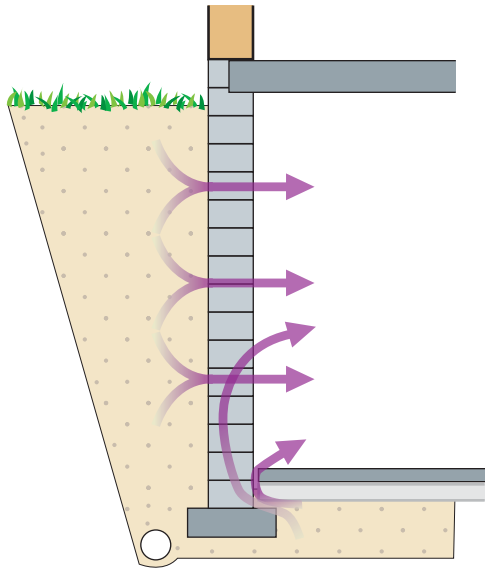
Kuva 1.3. Radonin vuotoreittejä, kellarillisessa rakennuksessa tai rintetalon alimmissa kerroksessa.
