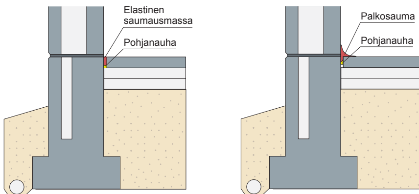
Kuva 6.1. Sokkelin ja laatan välisen sauman tiivistäminen.
